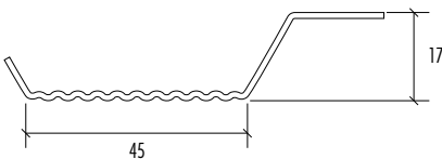
Resilient Bar
